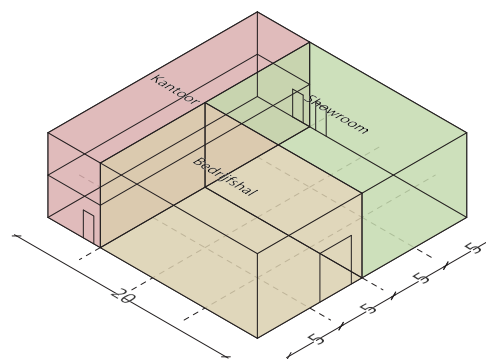
Configuratie voorbeeld 1 (formaat 20x20m)
